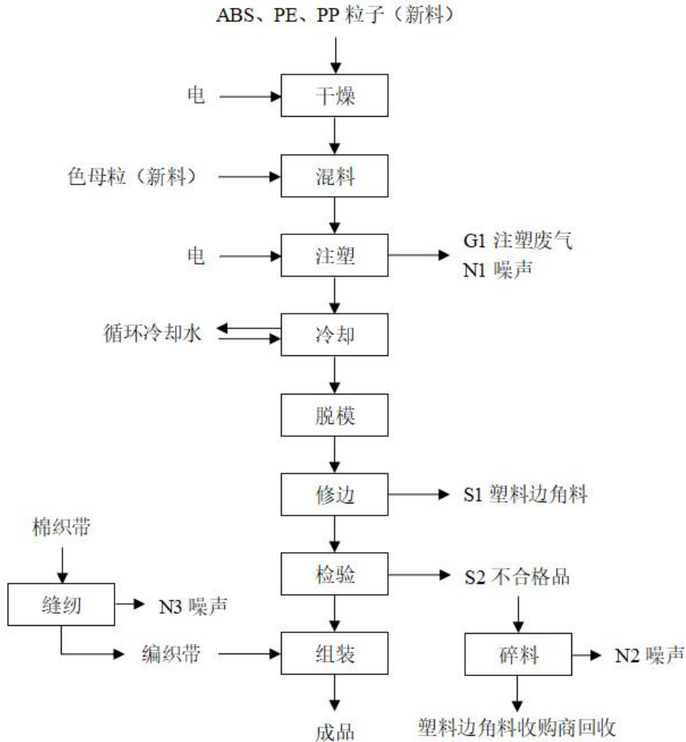
图 2-2 安全帽生产工艺流程图
