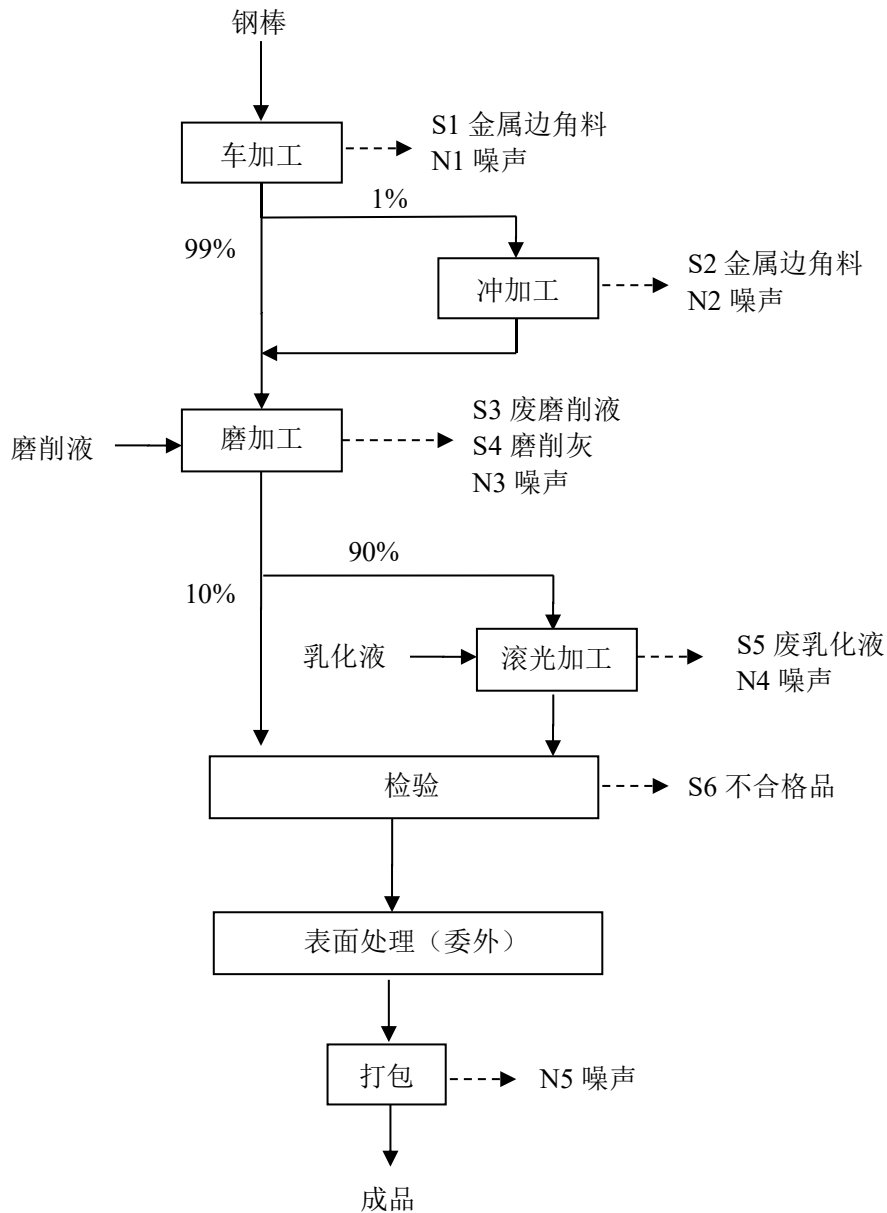
图 2-2 机械零部件生产工艺流程图
